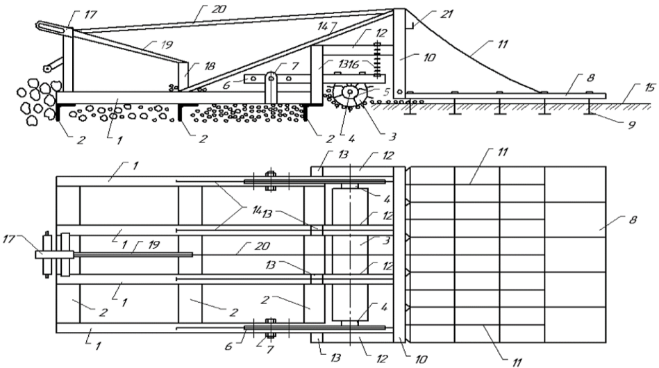
Рис. 1. Конструктивно-технологічна схема комбінованого ґрунтообробного агрегату
