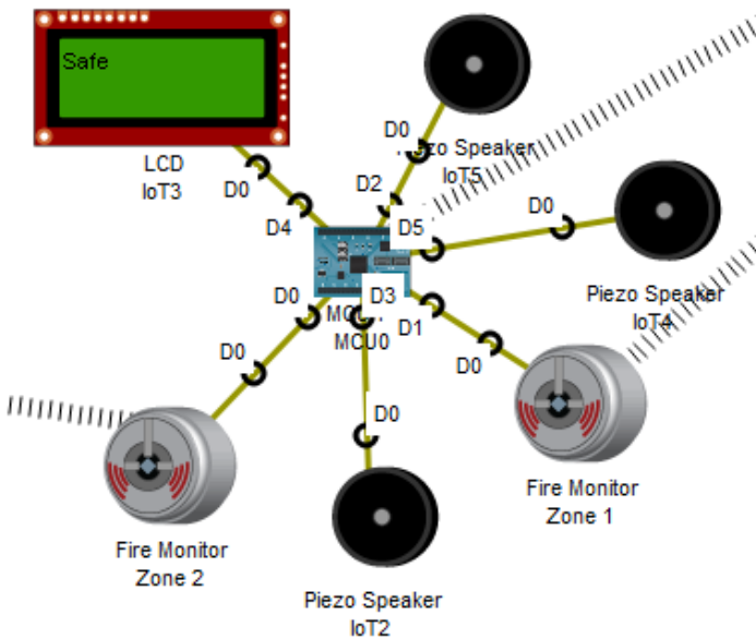
Рис. 2. Приклад протипожежної системи на базі технологій IoT
