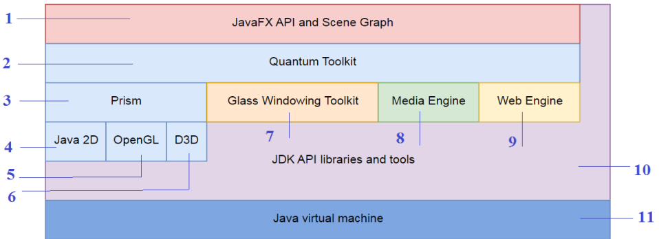
Рис.1. Архітектура платформи JavaFX [6]
